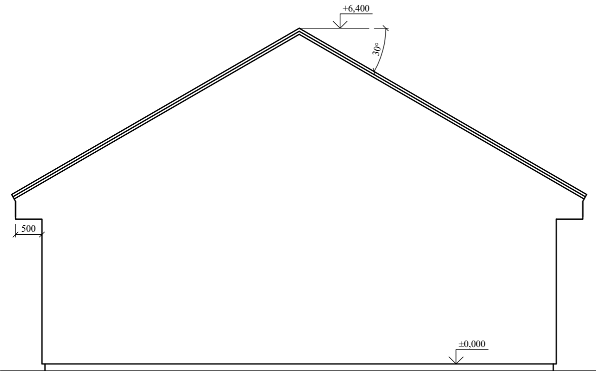
POHLED BOČNÍ
