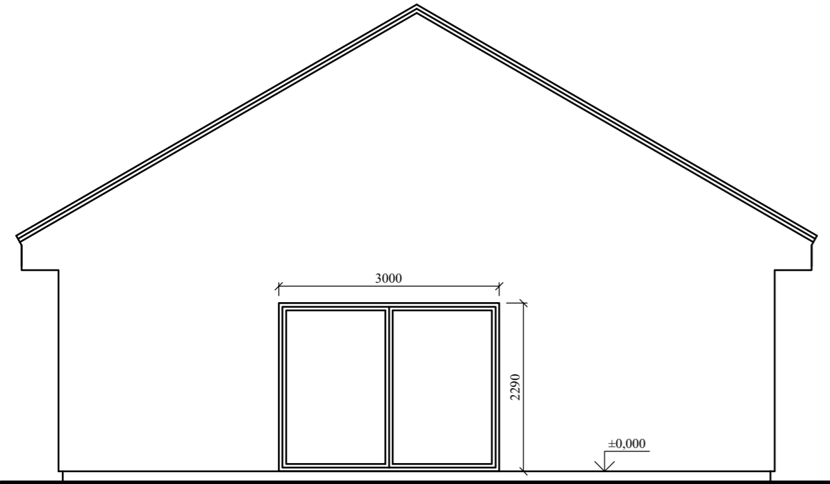
POHLED BOCNI
