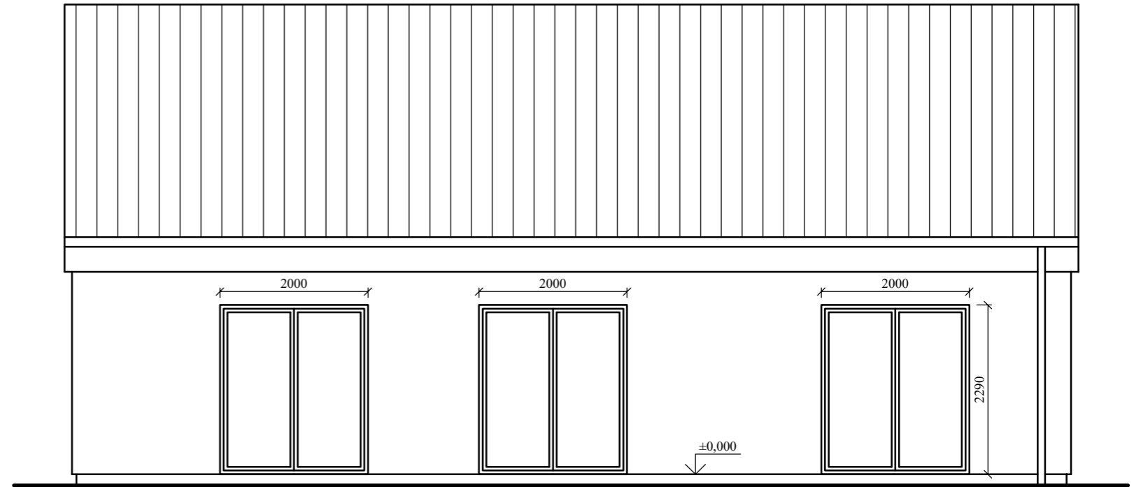
POHLED ZADNI
