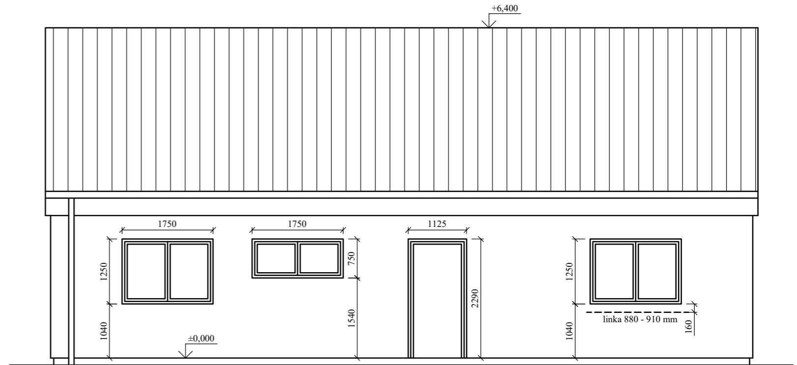
POHLED ČELNÍ
